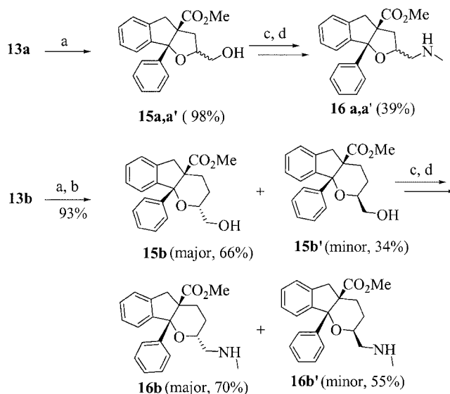
Scheme 2. Reagents and conditions: (a) m CPBA, CH_2Cl_2 ; (b) t BuOK, t BuOH; (c) Et 3 N, MsCl, DMAP, CH_2Cl_2 , 0 °C; (d) MeNH 2 , H 2 O, 120 °C, steel bomb
